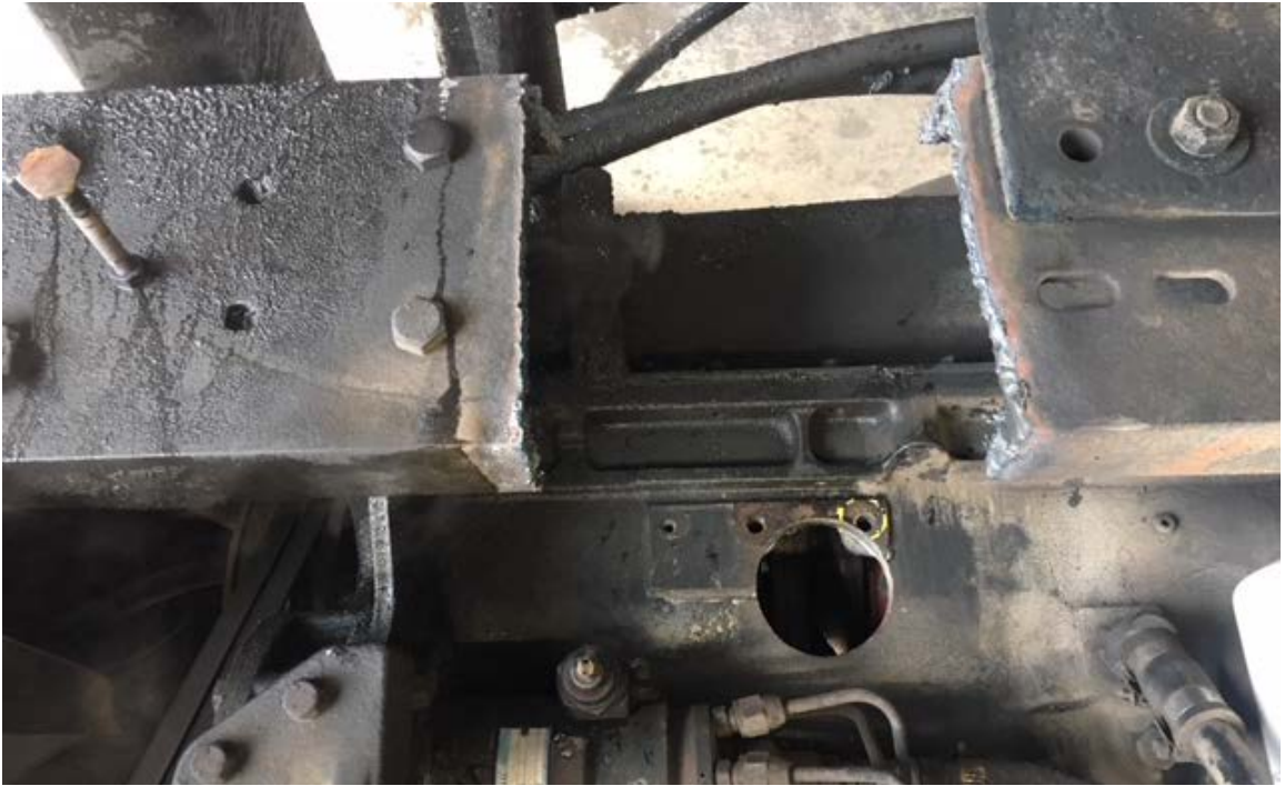
Figura 10. Foto de después, bloque del motor con agujero en un lado
